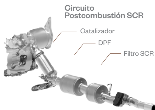
Tipos de sistemas de postcombustión
